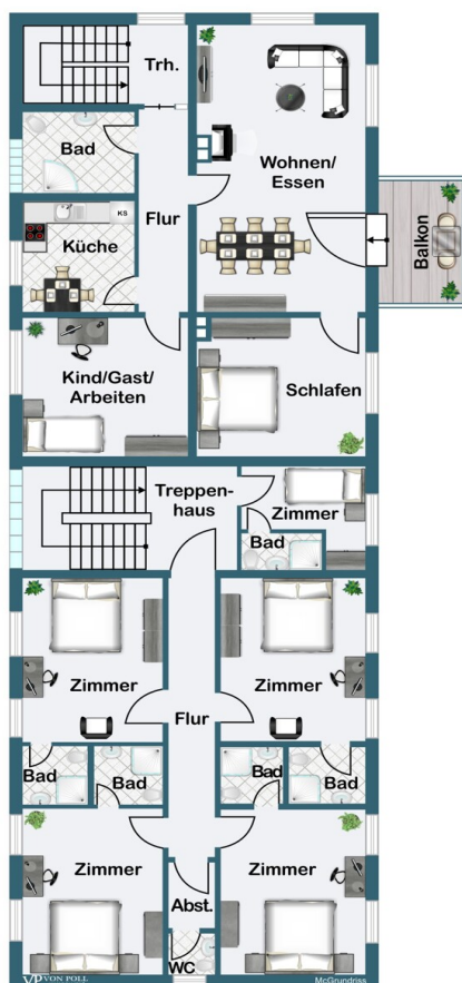
1. Obergeschoss
