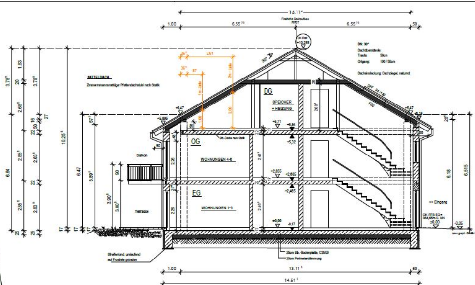
Schnitt B-B
