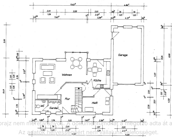
Erdgeschoß
