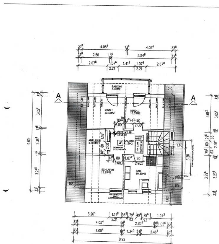
GRUNDRISS OBERGESCHOSS
