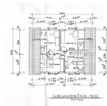
Grundriss Dachgeschoss
