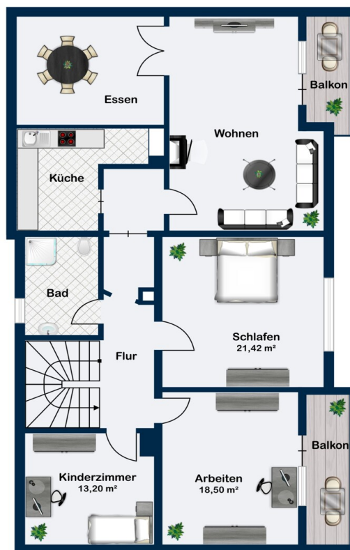
Obergeschoss
