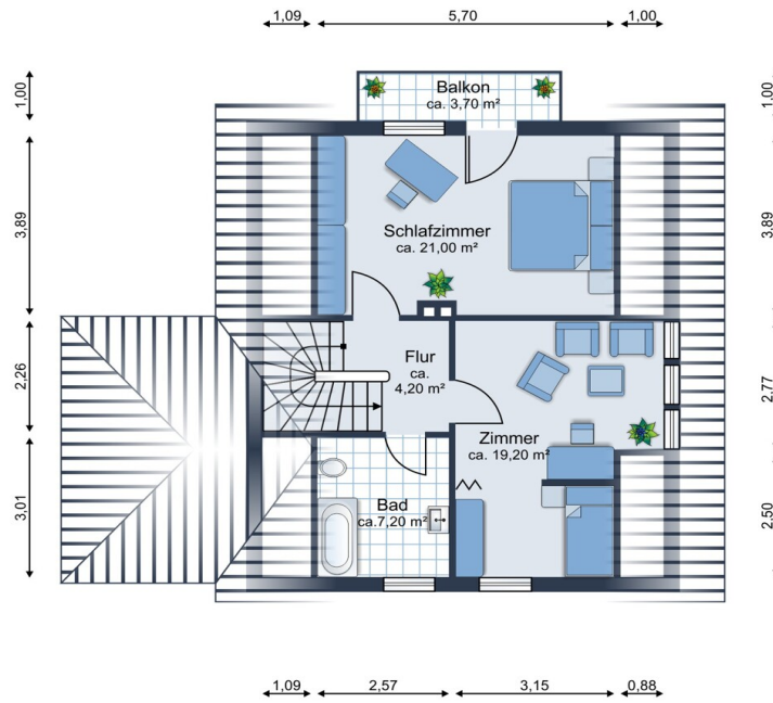
Dachgeschoss
