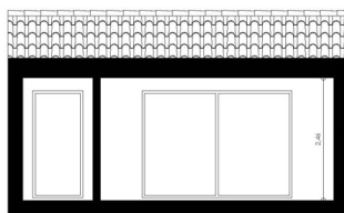
SECCIÓN D-D'
