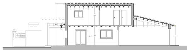
SECCION S-02 Escala 1:50
