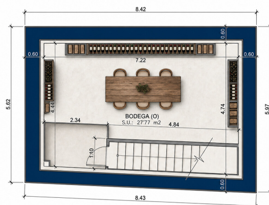
PLANTA SÓTANO
