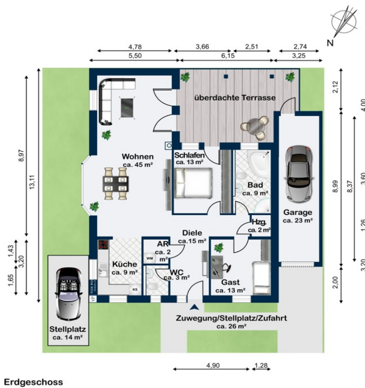
Erdgeschoss
