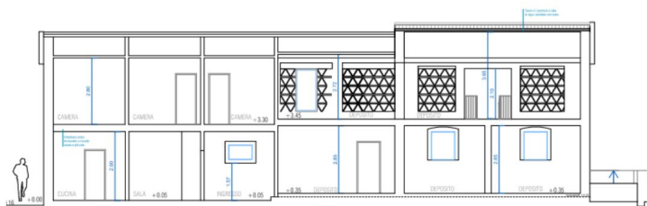
SEZIONE LONGITUDINALE AA'
