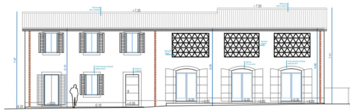
PROSPETTO FRONTE
