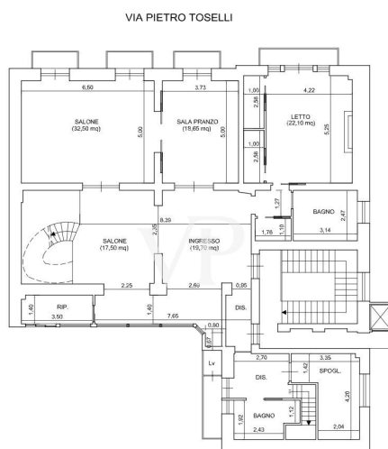
PIANTA PIANO TERZO H = 3.50 m
