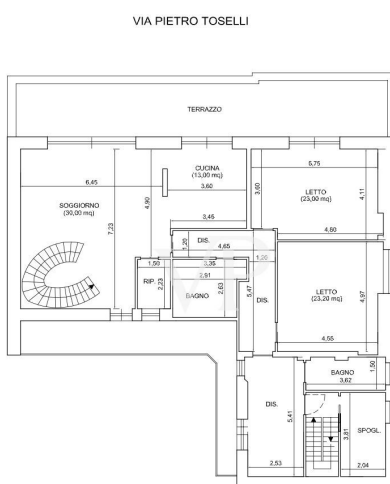
PIANTA PIANO QUARTO H = 3.45 m
