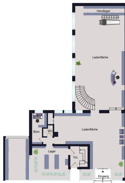
Erdgeschoss
