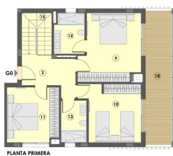
PLANTA PRIMERA
