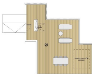
PLANTA SOLARIUM
