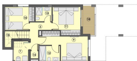
PLANTA SEGUNDA
