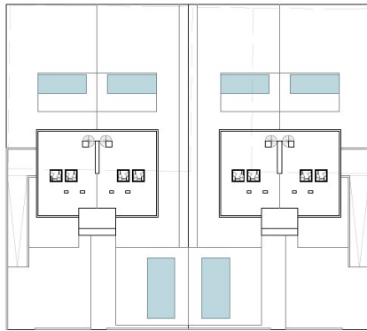
EMPLAZAMIENTO ECS 1/200
