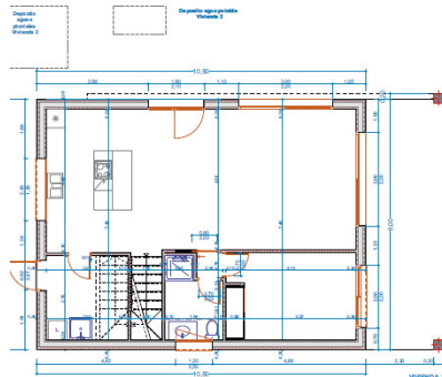
VIVIENDA 2 Planta Sót
