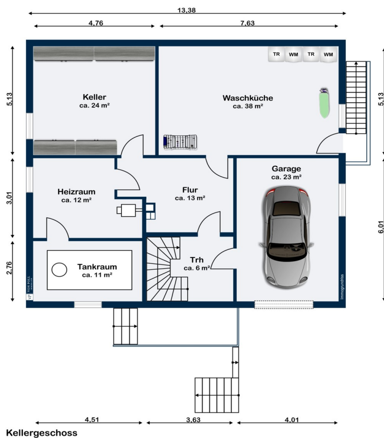
Kellergeschoss
