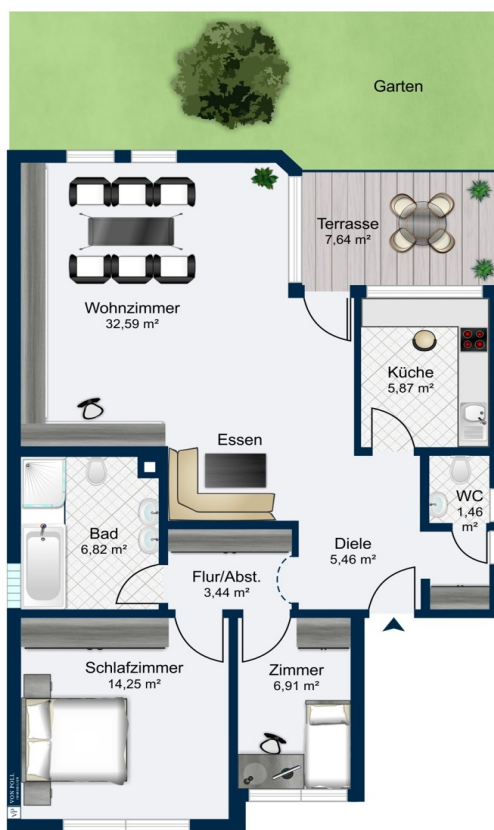
Erdgeschoss
