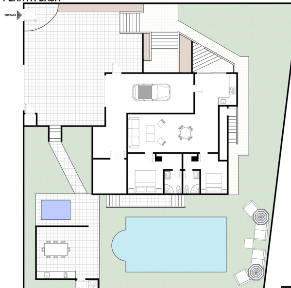
PLANTA BAJA
