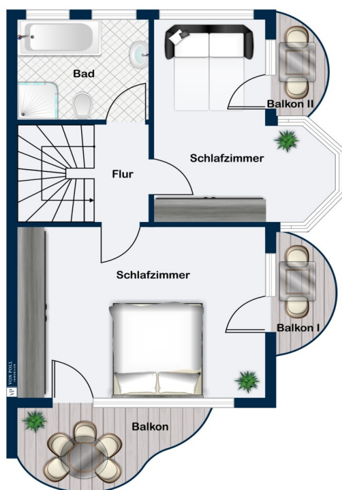
2. Obergeschoss
