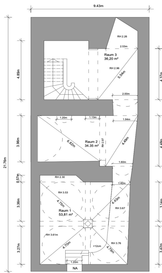
Grundriss KG 1:100
