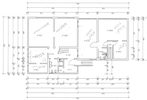
Derkere Str. 10 A Obergeschoss M 1 : 100
