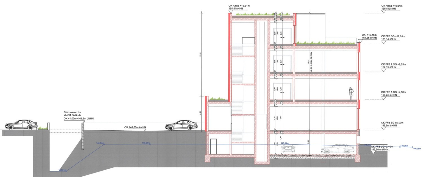
Schnitt C-C
