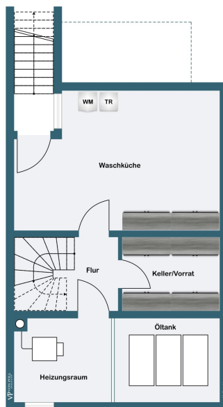
Kellergeschoss
