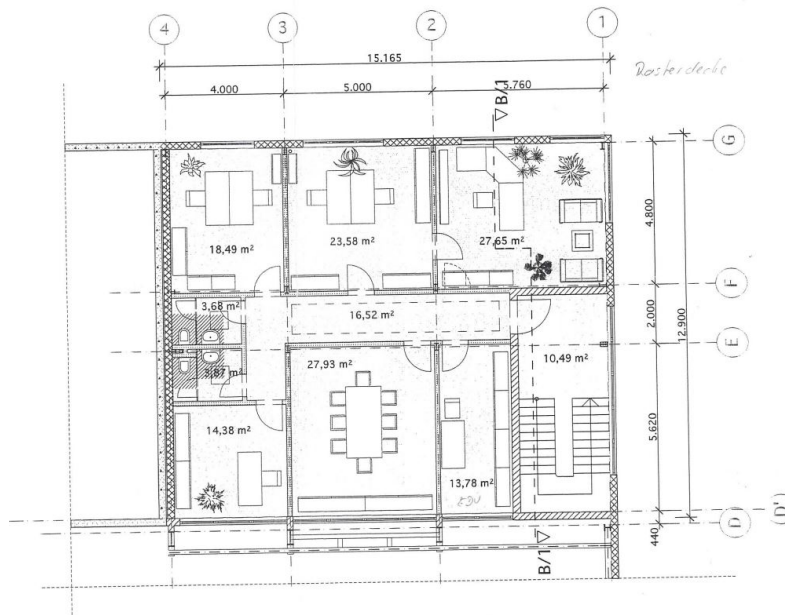
Grundriß Obergeschoß
