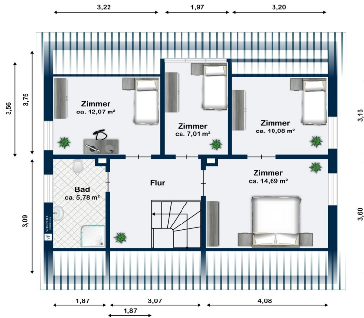
Dachgeschoss
