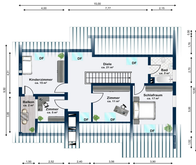
Dachgeschoss
