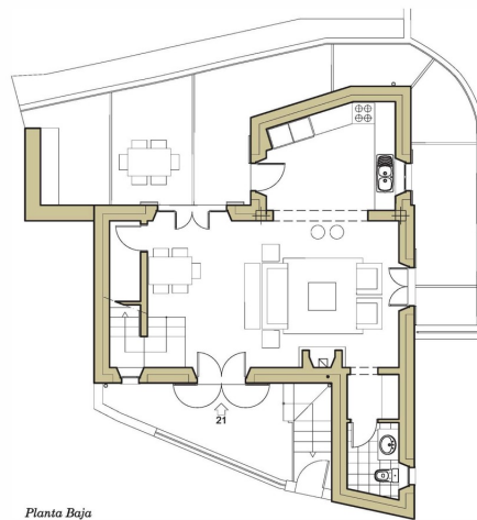
Planta Baja
