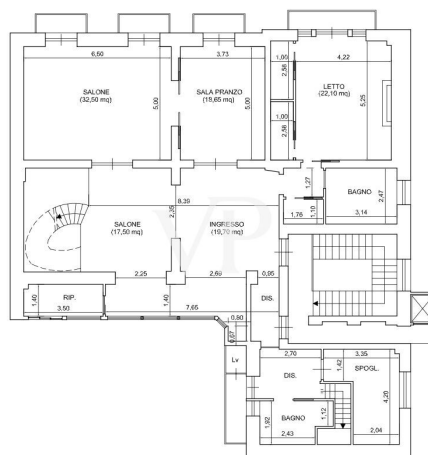
PIANTA PIANO TERZO H = 3.50 m
