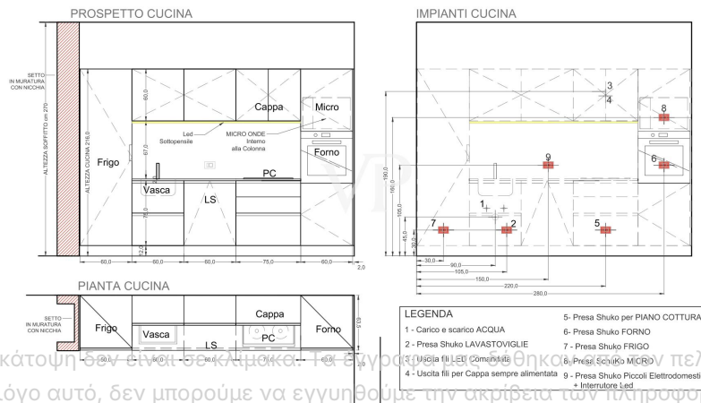
Scale: Client: 3/9-12-24 1:20 MATIERA IMPIANTI CUCINA (PERIIMPIANTO CUCINA) APPARTAMENTO 3 Piano Terreno
