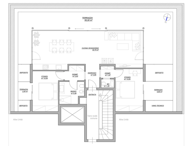
PLANIMETRIA APPARTAMENTO | 3° PIANO ATTICO
