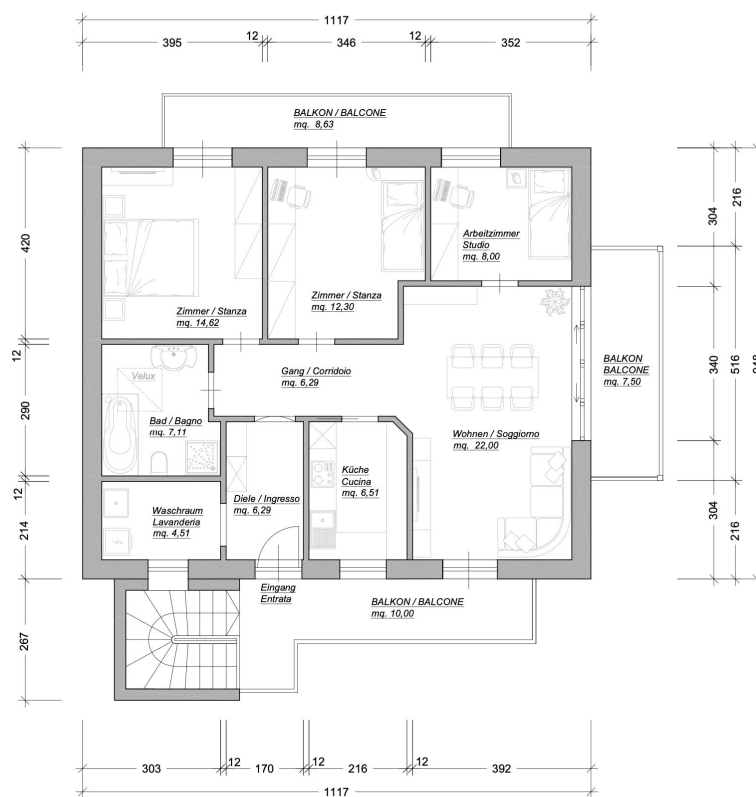
GRUNDRISS / PLANIMETRIA Bestand / Stato attuale
