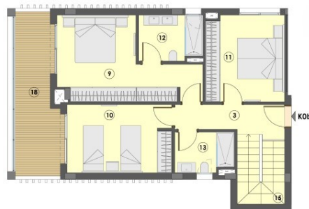
PLANTA PRIMERA
