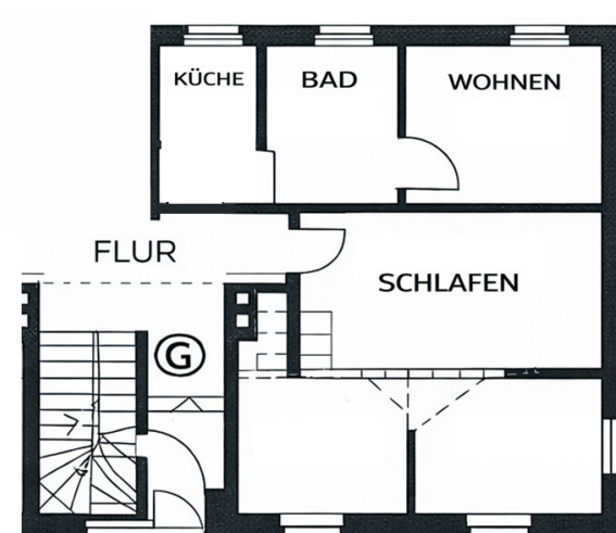
Grundriss Dachgeschoss
