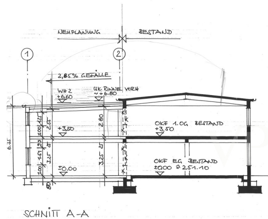
SCHNITT A-A
