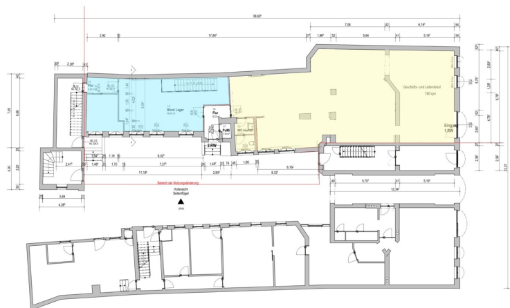
Erdgeschoss Neustädtischer Markt 5
