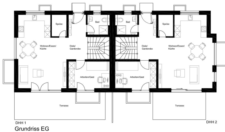
Grundriss EG
