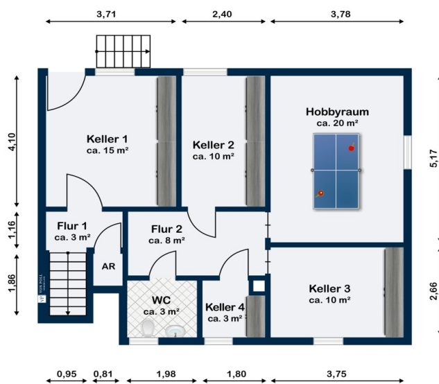
Kellergeschoss
