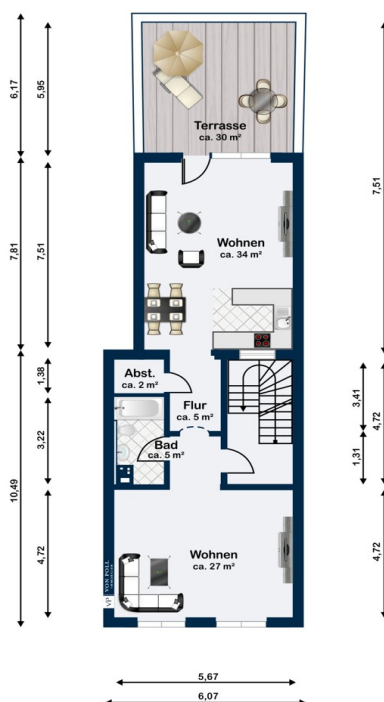
1. Obergeschoss
