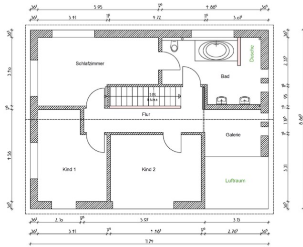
Grundriss Obergeschoss
