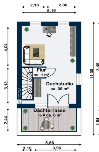
Dachgeschoss
