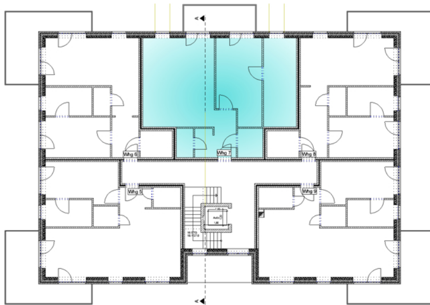
Obergeschoss
