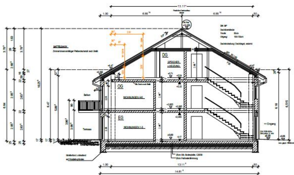
Schnitt B-B
