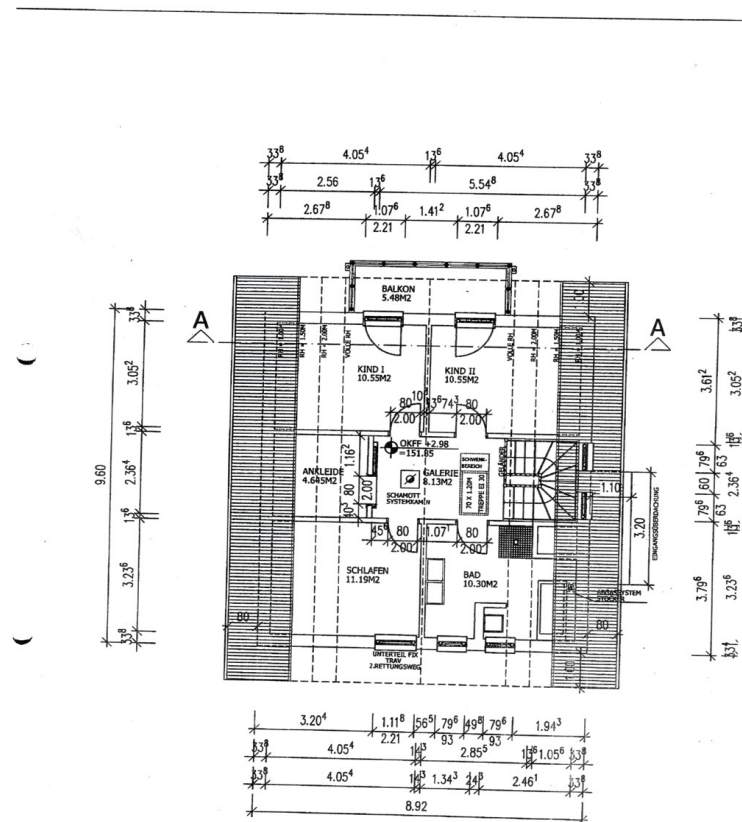
GRUNDRISS OBERGESCHOSS
