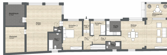
Erdgeschoss
