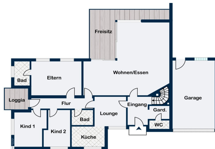
Erdgeschoss
